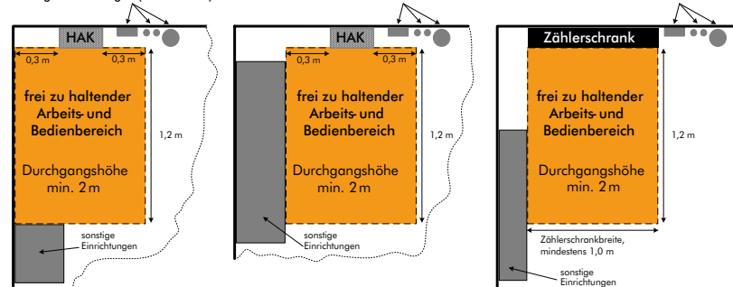
Bild 2 Ausführungsbeispiel einer Hausanschlusswand
