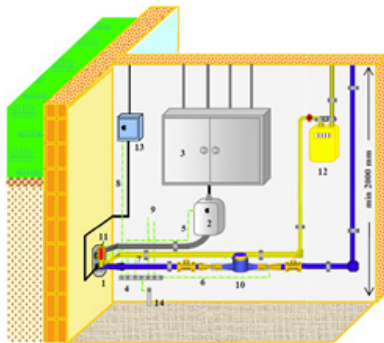
Bild 2 Ausführungsbeispiel einer Hausanschlusswand
